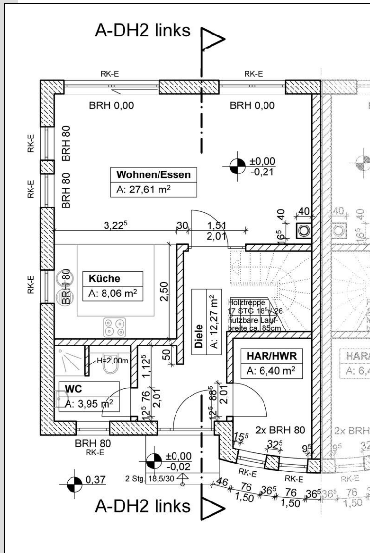
Grundriss EG
